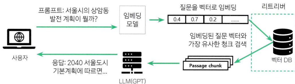
임베딩된 질문 벡터와 가장 유사한 청크를 검색하는 리트리버
