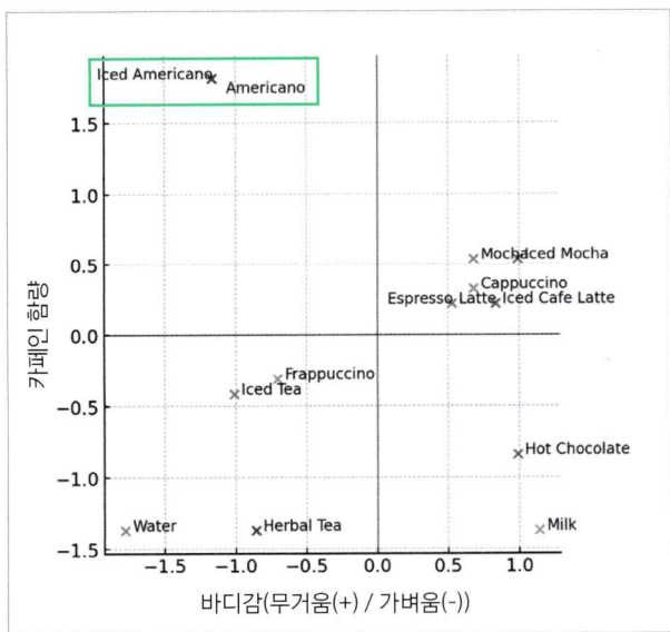
바디감과 카페인 함량을 기준으로 카페 음료 메뉴를 2차원 벡터 공간에 표현한 예
